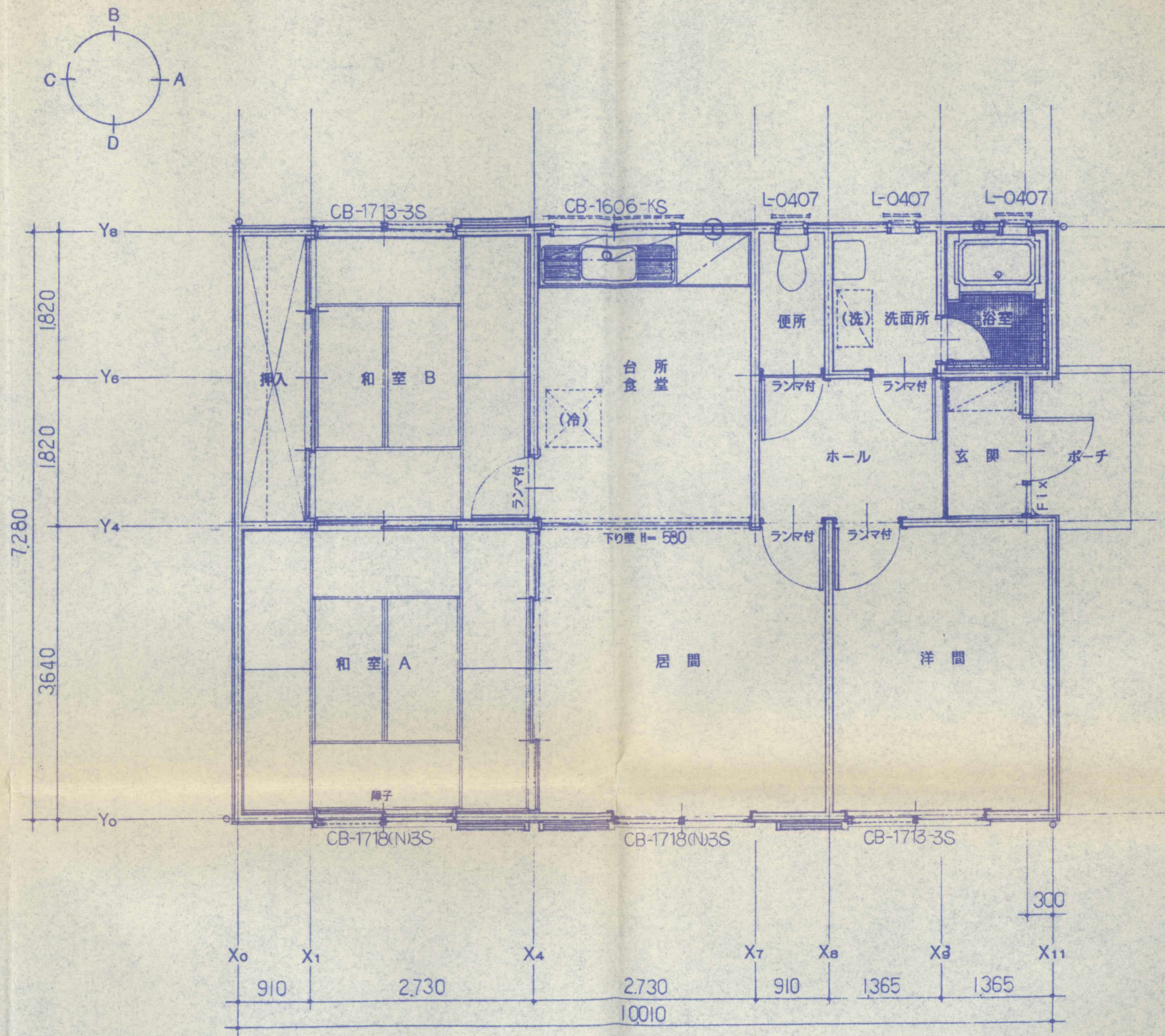
平面図
